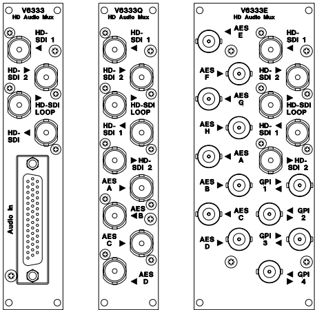
V16AR3AE V16AR3AG V16AR3AF
